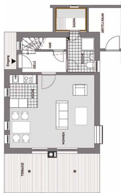
Grundriss Erdgeschoss
