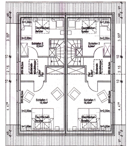
Dachgeschoss
