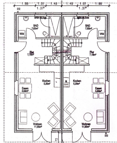
Erdgeschoss
